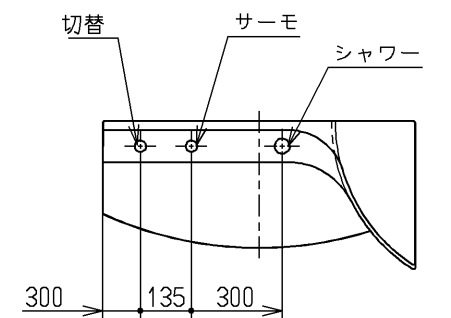
水栓取付け位置（フリー）
